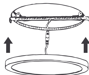
Instalación empotrada en orificio (Plafón)
